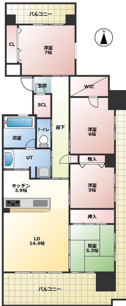
★間取り図★
